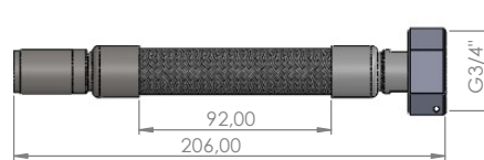
Kompensator DN16 z nakrętką 3/4 i króćcem do wspawania
