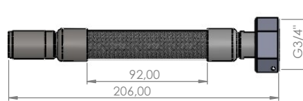
Kompensator DN16 z nakrętką 3/4 i króćcem do spawania
